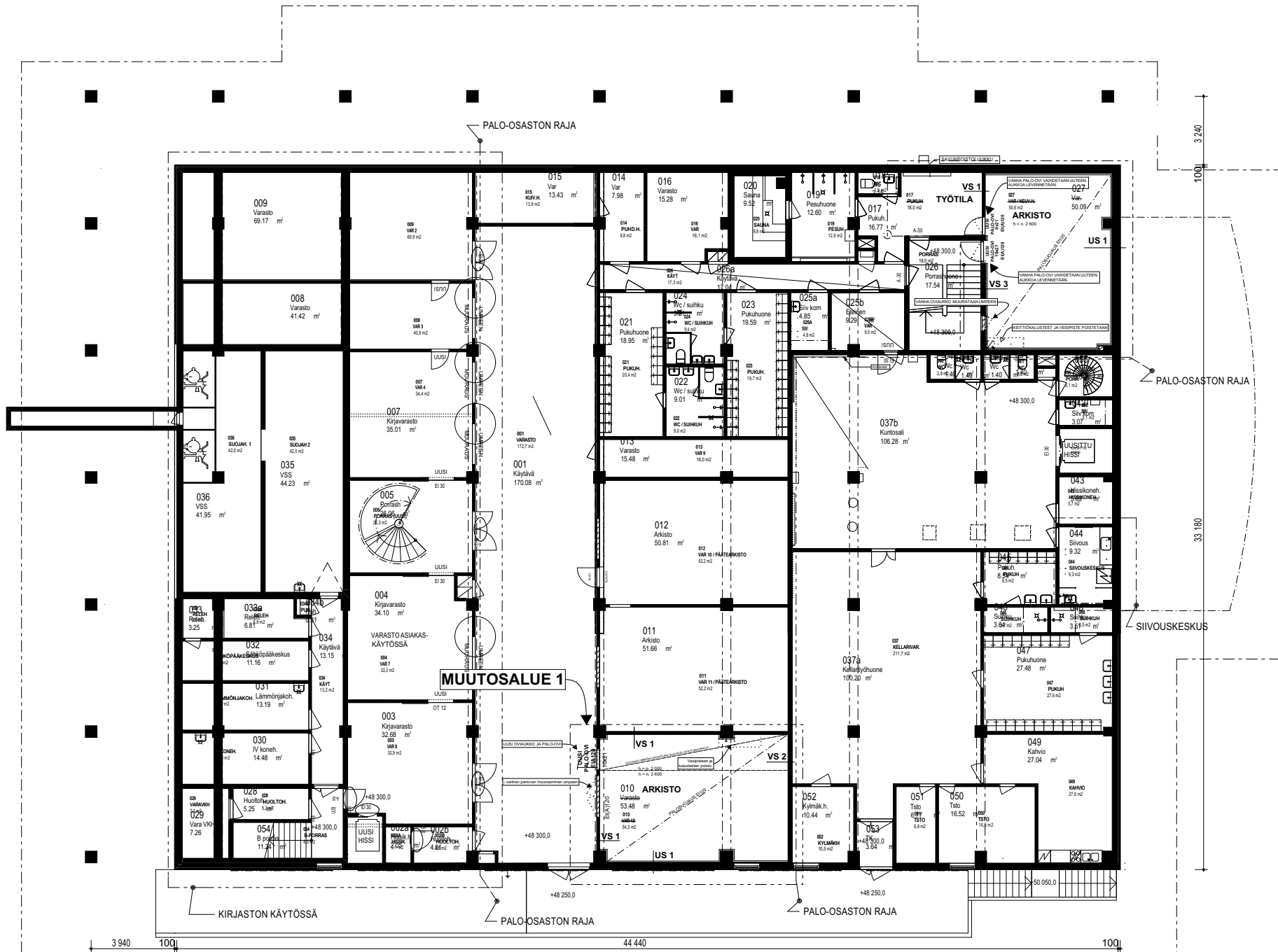
Pohjapiirustus kellarikerros
